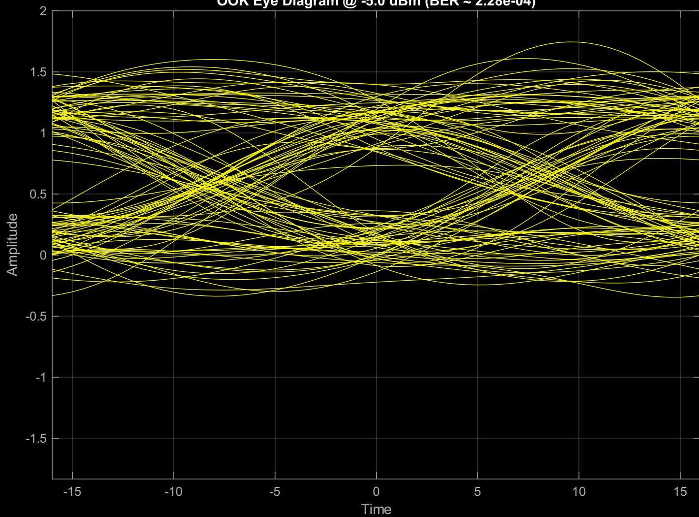
OOK Eye Diagram @ -5.0 dBm (BER \approx 2.28\text{e-}04 )
